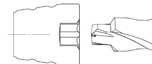
Spitzenwinkel 180° oder 170°
